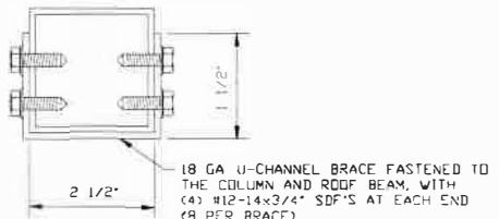
BRACE SECTION SCALE: NTS
